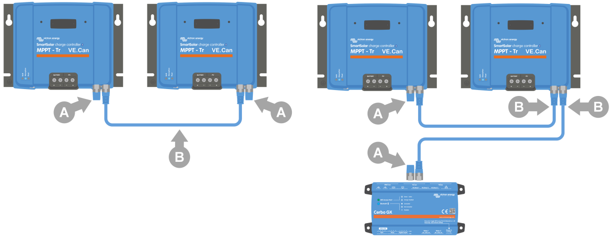
A: VE.Can-pääteiliitin - B: RJ45 UTP -kaapeli.
