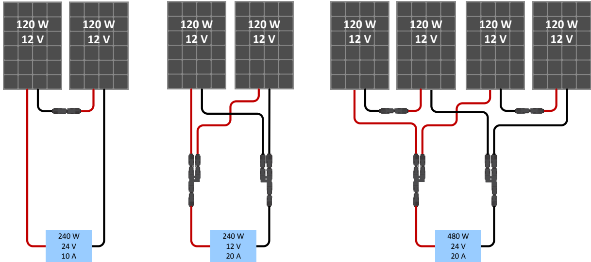
Esimerkkejä sarjaan-, rinnan- ja sarjaan/rinnankytyistä aurinkopaneeliryhmistä.
