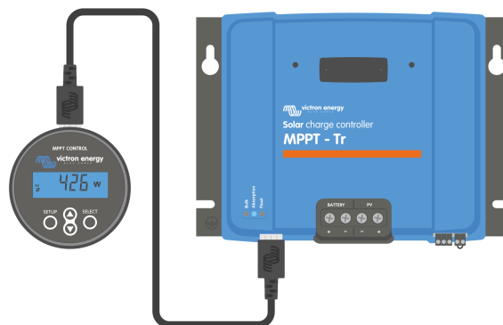
Liitä näyttö lataussäätimeen VE.Direct-kaapelilla
