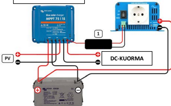
Kuva 6: Victron-inverterimallit Phoenix 12/180, 24/180, 12/350, 24/350, Phoenix Inverter C -mallit ja MultiPlus C -mallien liitäntä edellyttää liitäntäkaapelin (1) käyttöä: " Inverting remote on-off cable " (tuotenumero ASS030550100)
