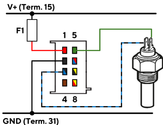
Isolierte Masse-Rückleitung
